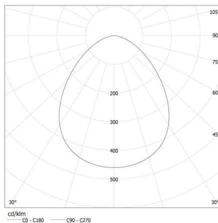
KANLUX S.A. (kat 25781) IVIAN LED 4,5W SN-WW / Krzywa rozsyłu światła (biegunowo)
