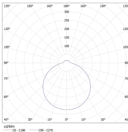
KANLUX S.A. (kat 28720) BIGGE LED 42W-WW-O / LDC (Polar)
