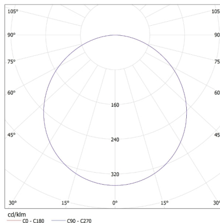
KANLUX S.A. (kat 29821) BLINGO LED48W 6060 NW / LDC (Polar)
