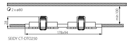
SEIDY CT-DTO250
