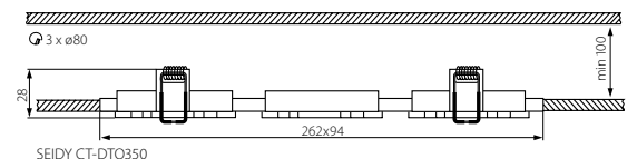
SEIDY CT-DTO350
