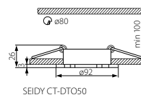
SEIDY CT-DTO50
