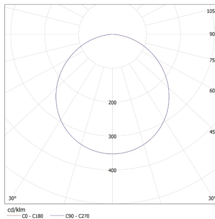
KANLUX S.A. (kat 27221) ROUNDA V2LED6W-NW-SN / LDC (Polar)
